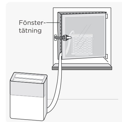
Exempel på en installerad PortaSplit-fönstertätning.
